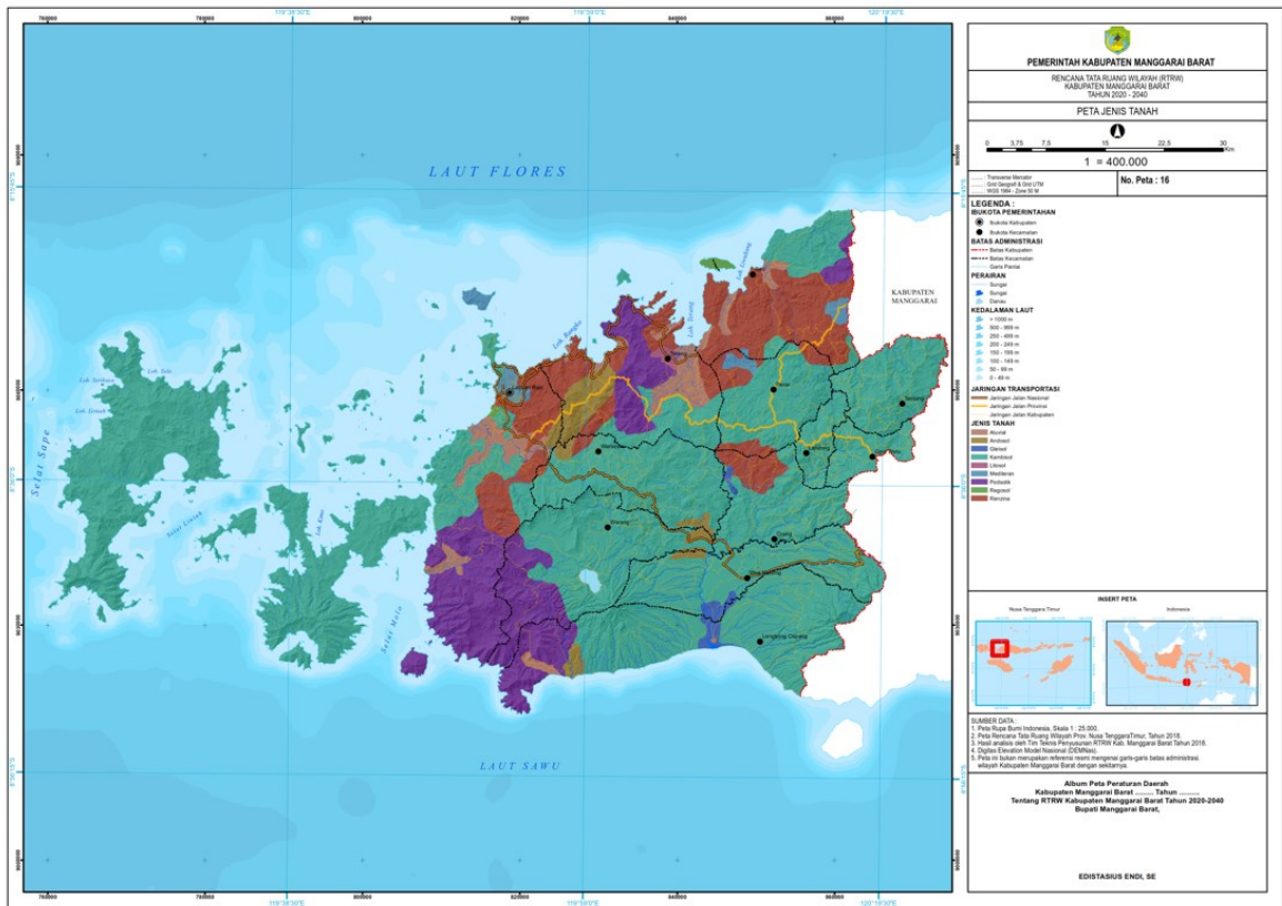
Gambar 2. 5. Peta Jenis Tanah Kabupaten Manggarai Barat
