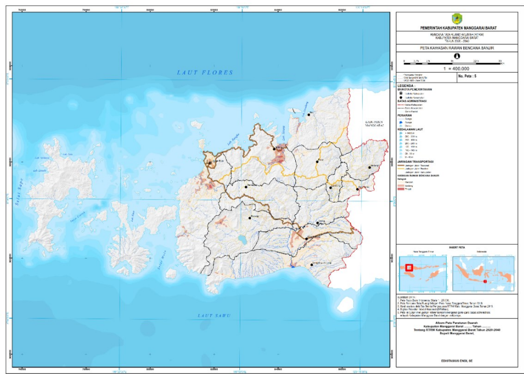
Gambar 2. 12. Peta Tingkat Kerawanan Bencana Banjir Kabupaten Manggarai Barat Sumber: Dokumen RTRW Kabupaten Manggarai Barat, 2023
