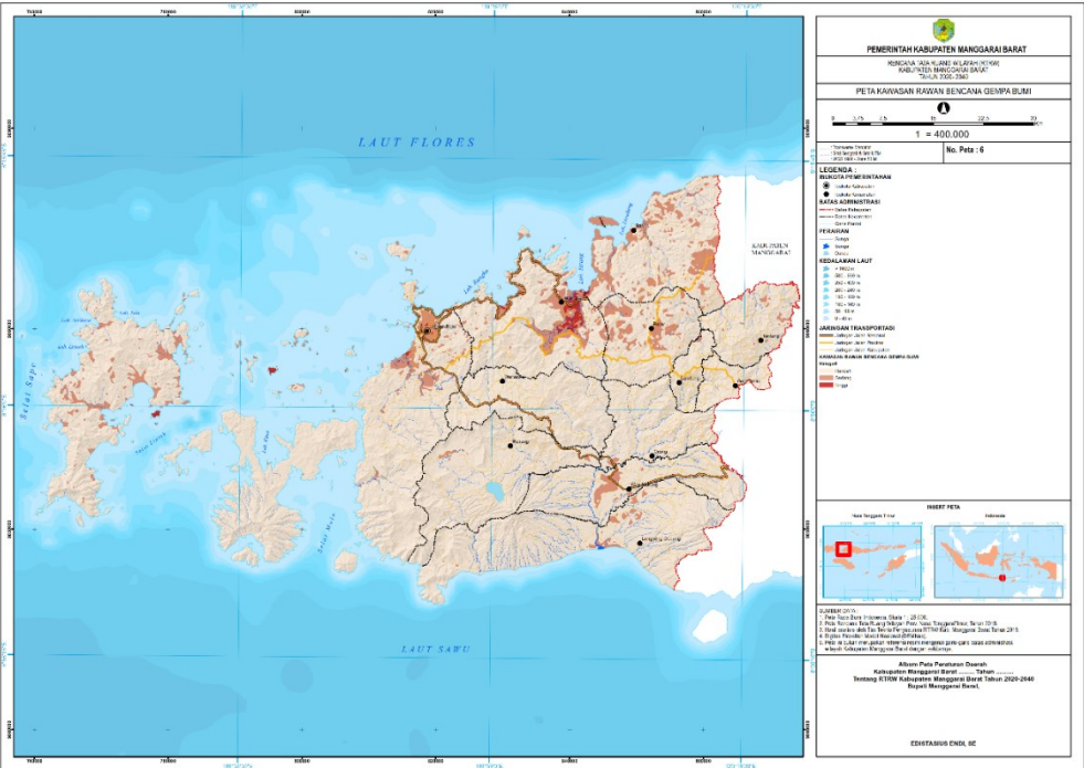
Gambar 2. 9. Peta Kerawanan Gempa Bumi Kabupaten Manggarai Barat Sumber: Dokumen RTRW Kabupaten Manggarai Barat, 2023
