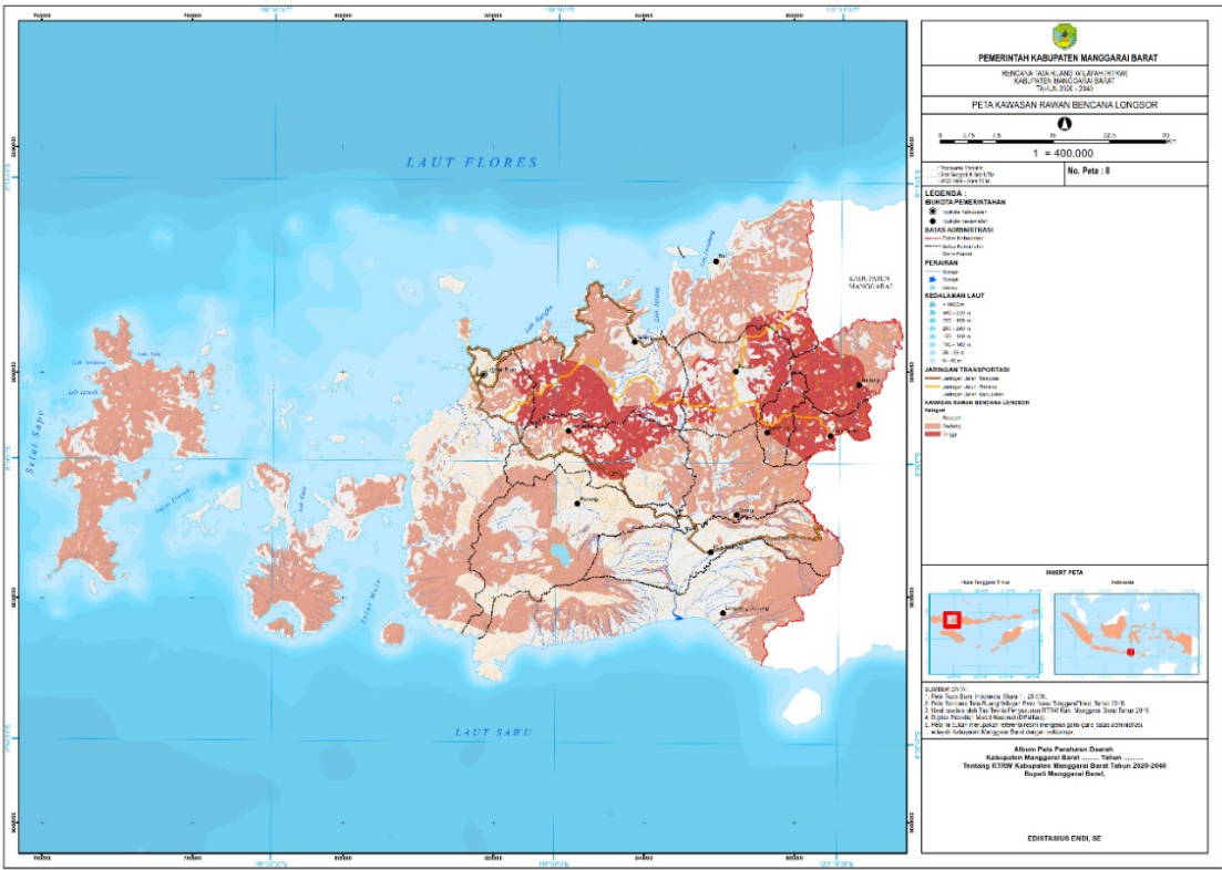
Gambar 2. 11. Peta Tingkat Kerawanan Longsor di Kabupaten Manggarai Barat
